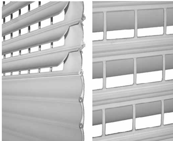
JalouRoll combine avec un tablier volet roulant et fonction BSO
